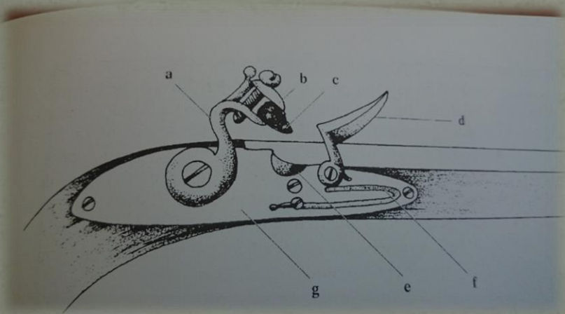
Nákres zbrane
